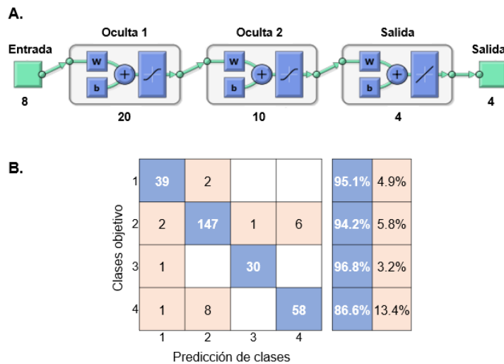
Figura 4-3 Resultado de la clasificación de edad A. Red neuronal multicapa B. Matriz de confusión
