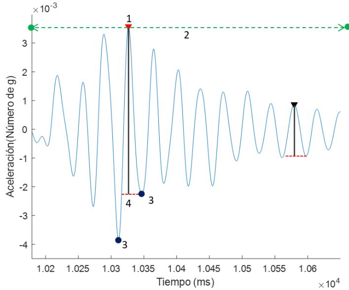
Figura 3-12 Ejemplo de medición de prominencia en la señal de una pisada
