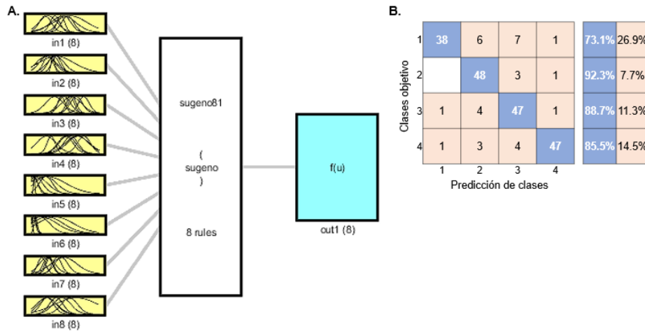
Figura 4-8 Resultado de la clasificación de IMC A. Clasificador neurodifuso adaptable con modificadores lingüísticos B. Matriz de confusión
