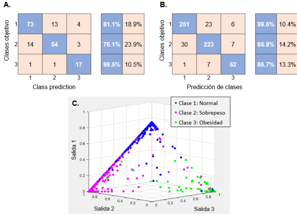
Figura 4-16 Resultado de la clasificación por IMC con red neuronal con función de activación softmax A. Matriz de confusión de datos de prueba B. Matriz de confusión de todos los datos C. Gráfico 3D
